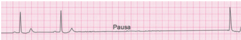
Fig. 8.12: Pausa sinusal
