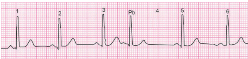
Fig. 8.1: Latidos prematuros
