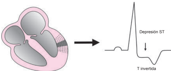
Fig. 7.20: Isquemia
