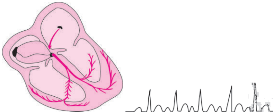
Fig. 8.20: Taquicardia auricular
