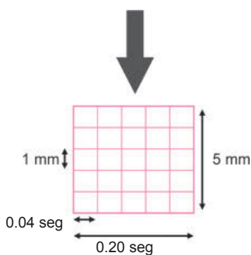
Fig. 6.2: La altura se mide en milímetros (mm) y la anchura en milisegundos (ms). Gráfica de voltaje vs tiempo.
