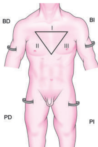
Fig. 4.1: Derivaciones
