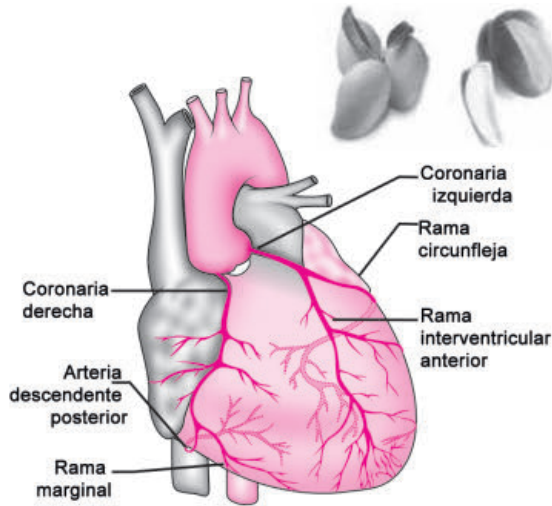
Fig. 7.27: Corazón
