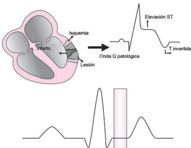
Fig. 7.19: Segmento ST
