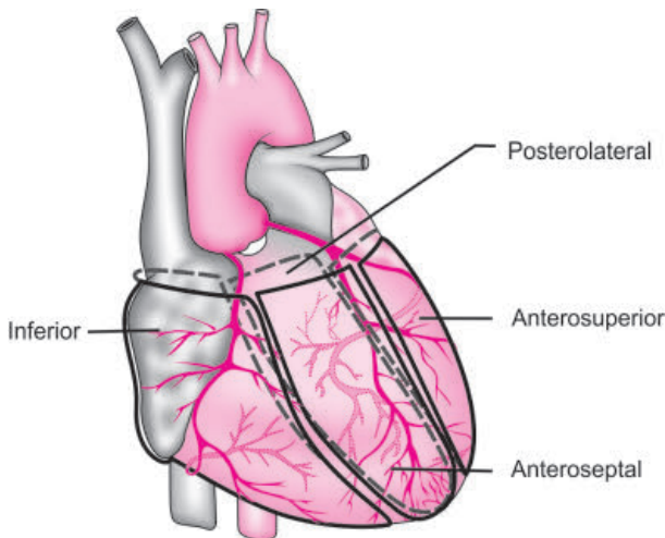
Fig. 7.28: Cuadrante VI
