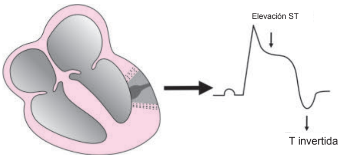
Fig. 7.21: Lesión
