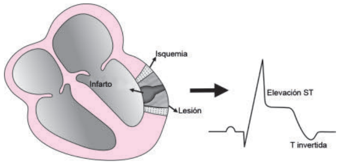
Fig. 7.22: Infarto
