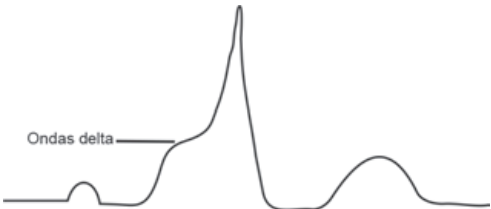
Fig. 8.32: Ondas delta
