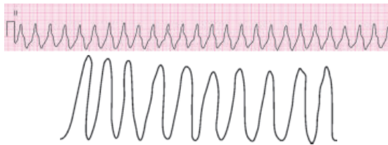
Fig. 8.28: Taquicardia ventricular
